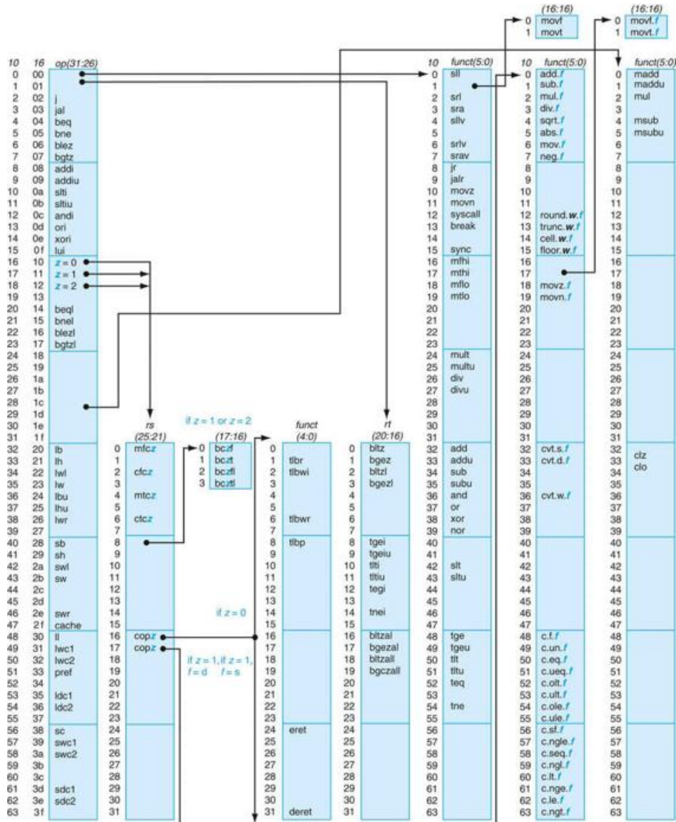
FIGURE A.10.2 MIPS opcode map.
